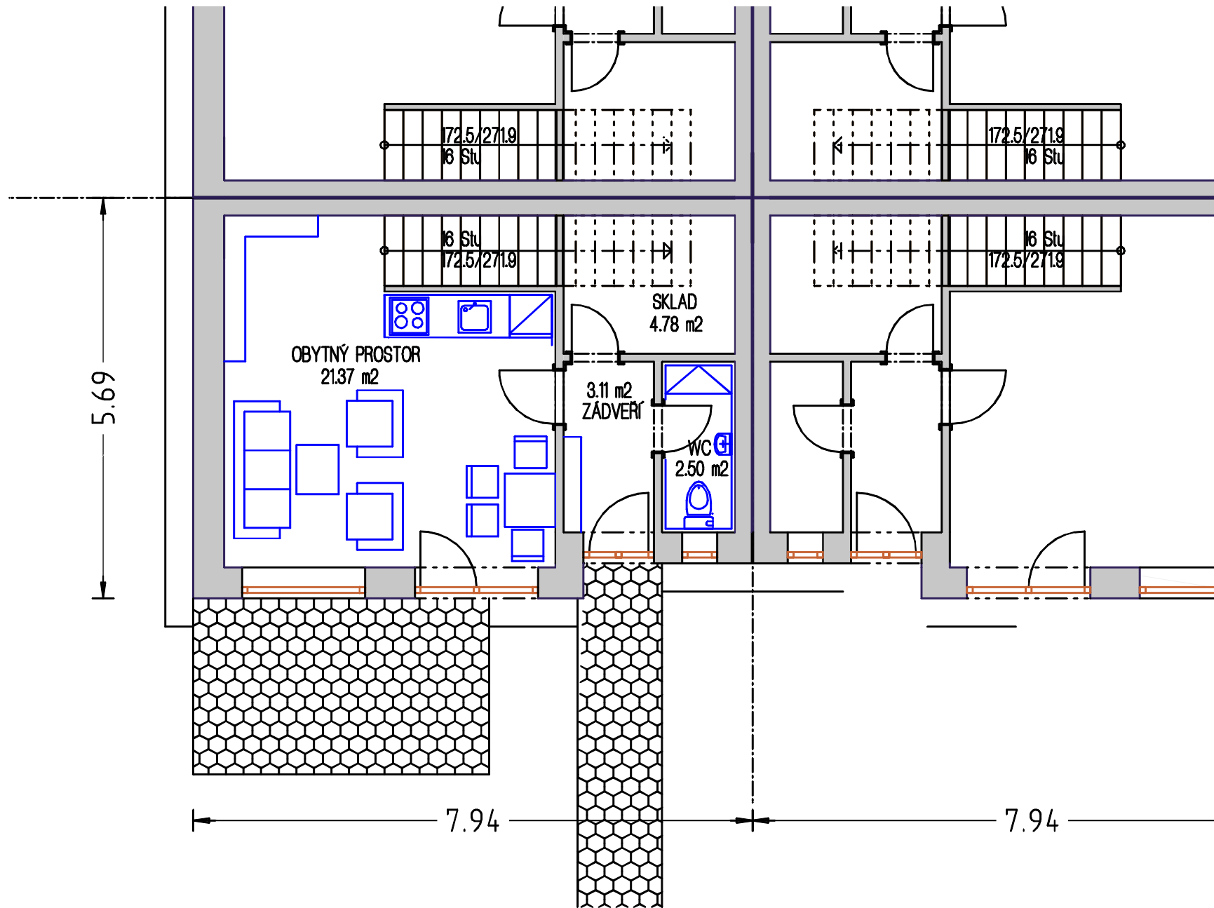
Půdorys I.NP
